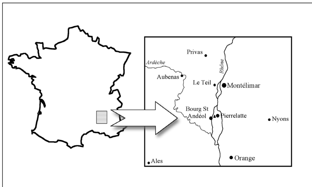
Fig. 1 : Localisation géographique du secteur étudié. La coupe de Pierrelatte est signalée par le symbole ▲.
