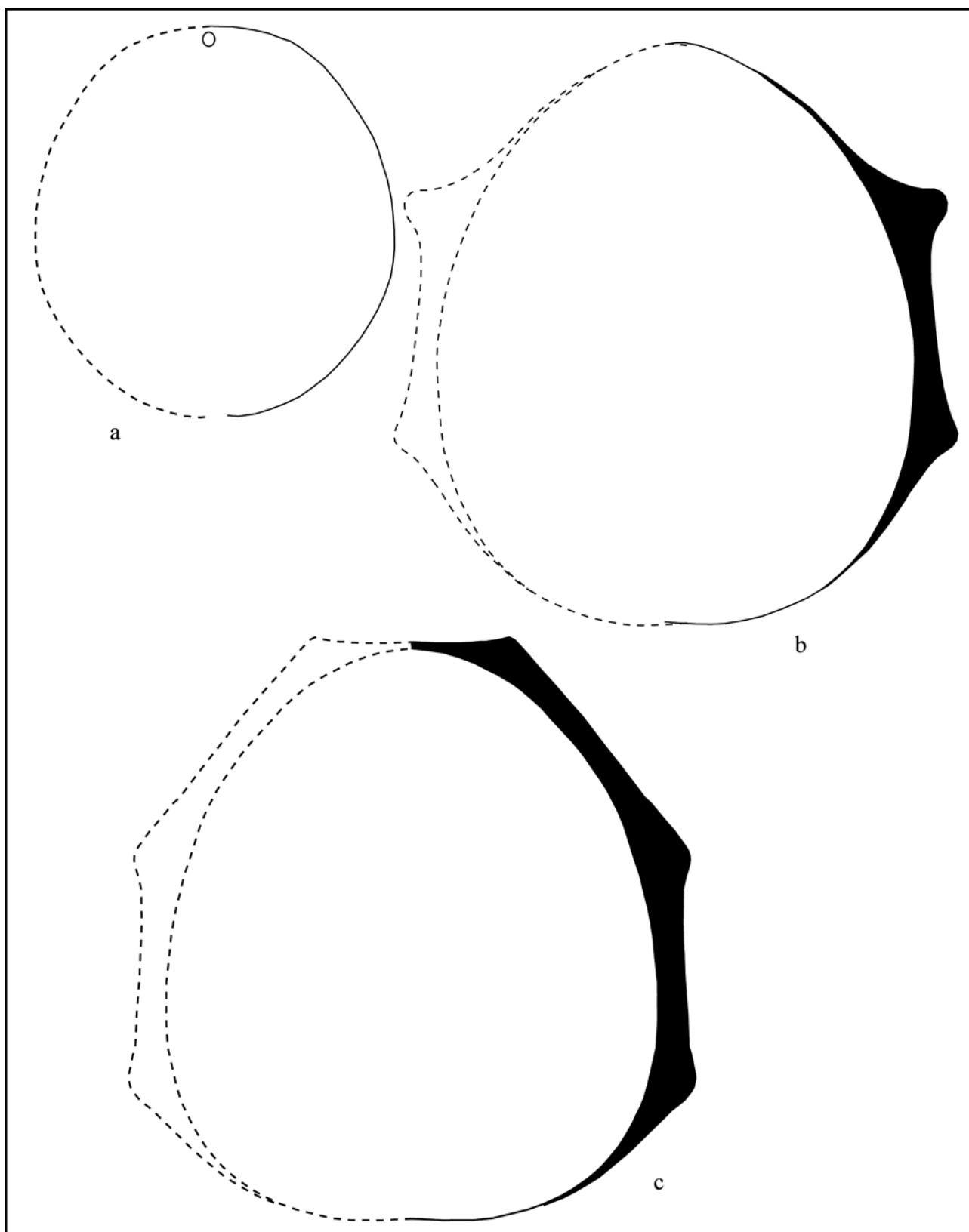
Fig. 5: Section du tour de Lythancylus renatae sp. nov., paratype, éch. MHNG 38874, X 0,87
