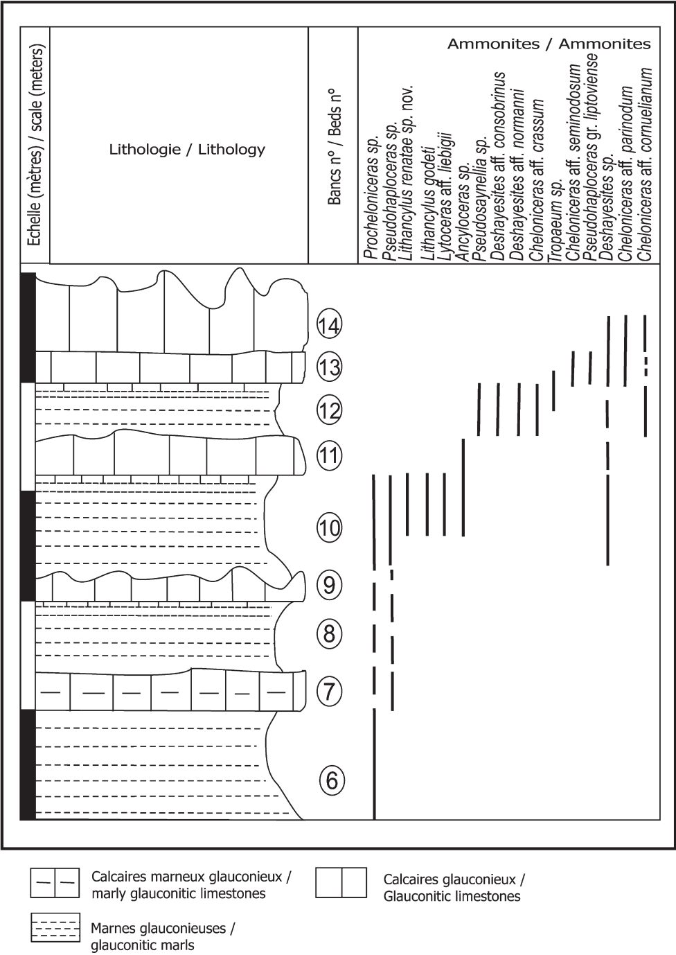
Fig. 2: Coupe stratigraphique de Pierrelatte.
