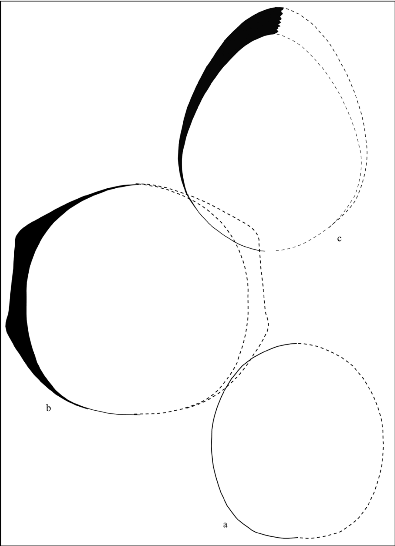
Fig. 4: Section du tour de Lythancylus renatae sp. nov., holotype, éch. MHNG 38873, X 0,86
